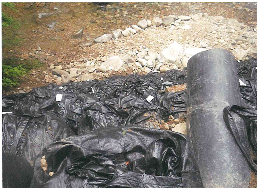
若樺榎谷林道（下） 令和3年6月15日 崩壊箇所仮復旧完了 路面から下方向撮影
