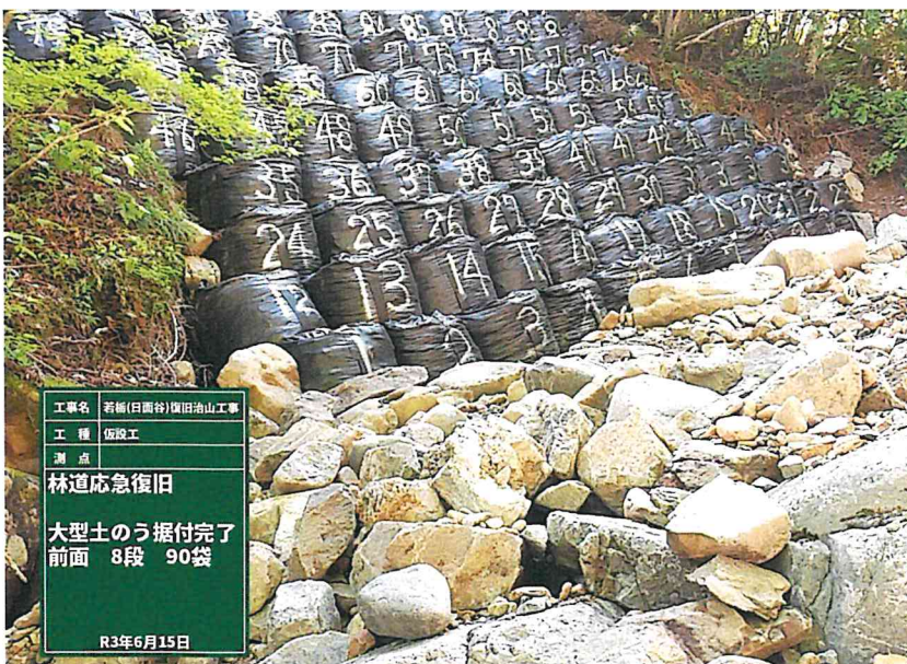
若瀬榎谷林道（下） 令和3年6月15日 崩壊箇所仮復旧完了 下流側から撮影
