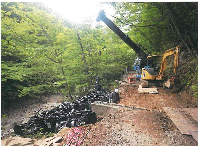
若栃榎谷林道（下） 令和3年6月10日 崩壊箇所仮復旧状況
